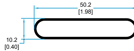
6100 LAMA MALLORQUINA.
