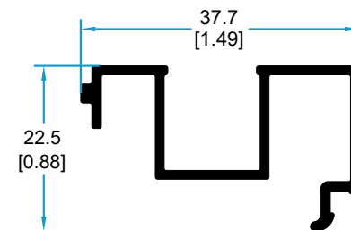
6031 JUNQUILLO MALLORQUINA.
