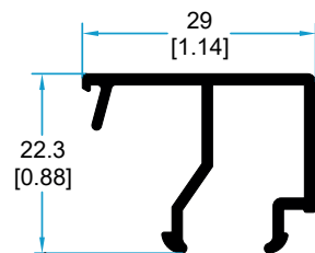
6017 JUNQUILLO HUECO.
