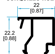
6018 JUNQUILLO HUECO.
