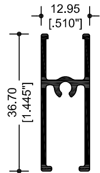
9956 CABEZAL Y ZOCLO
