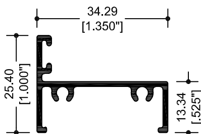
33087 MARCO PARA PUERTA
