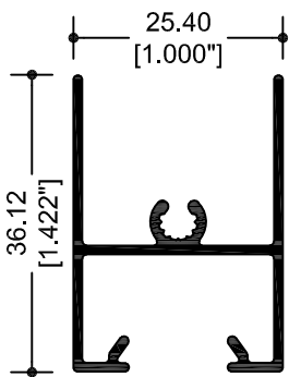
67836 CABEZAL
