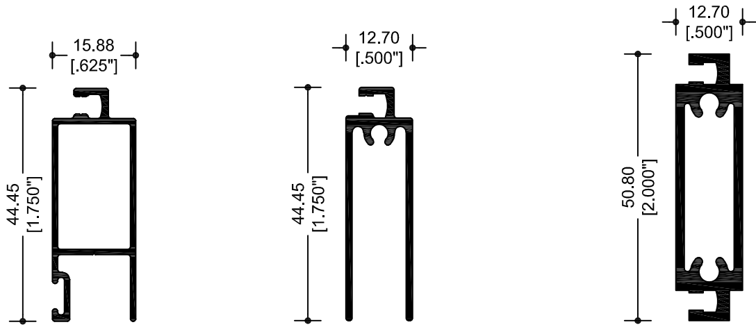
66534 CERCO MOSQUITERO
