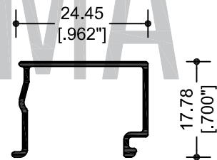
69890 JUNQUILLO CUADRADO SENCILLO (6mm)
