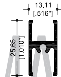
11203 INTERMEDIO PARA CUADRÍCULA
