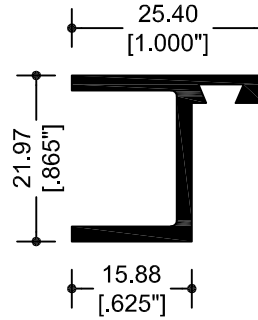
7102 BATIENTE
