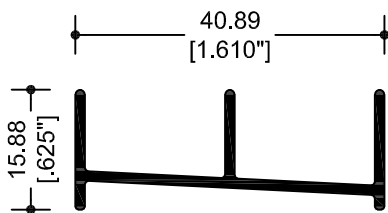
10198 RIEL INFERIOR
