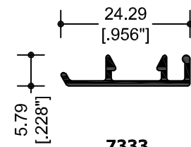
7333 MOSQUITERO
