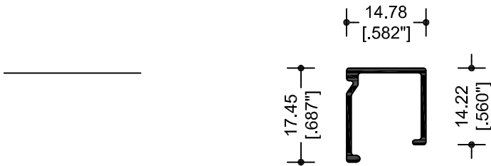
36370 JUNQUILLO
