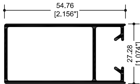
9236 CERCO CHAPA
