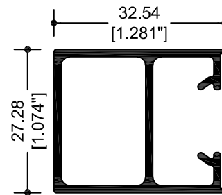
67843 CERCO VENTANA
