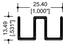
63329 GUÍA
