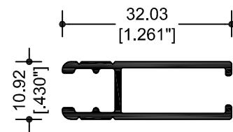
53358 ZAPATA
