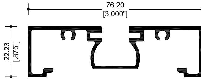
69105 BOLSA CORTA SIN TEMPLE Y TEMPLE 05
