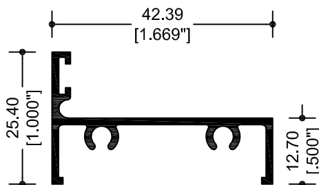
68550 MARCO PARA PUERTA
