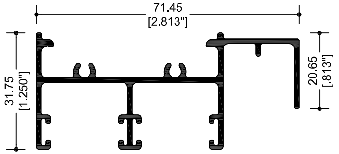
27819 CABEZAL MOS. CORREDIZO
