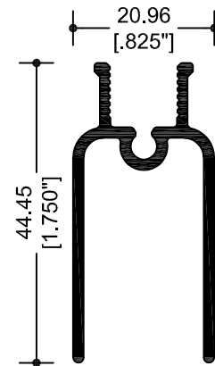
7108 CABEZAL Y ZOCLO
