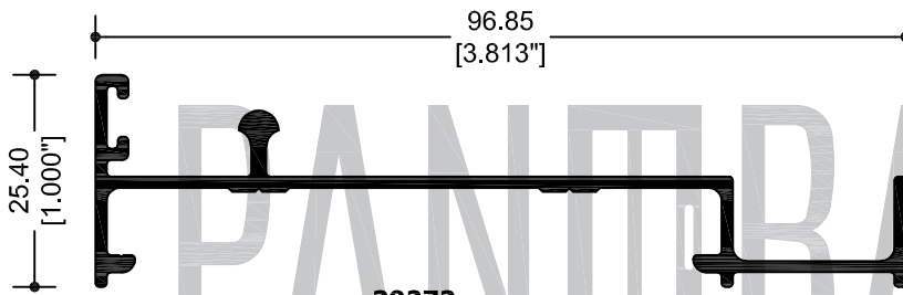
39272 RIEL PARA MOS. EXT. CORREDIZO
