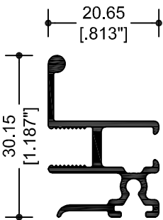
10571 CERCÓ MÓVIL
