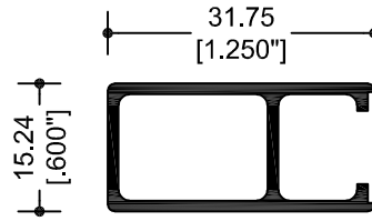
8320 CERCO VENTANA
