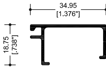
28939 JUNQUILLO
