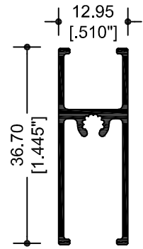
11044 CABEZAL Y ZOCLO
