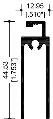
7104 MOSQUITERO
