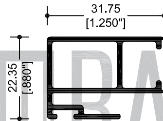
39954 TRASLAPE VENTANA
