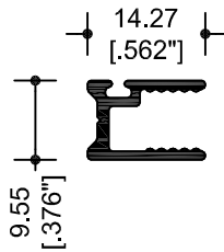
10574 CERCÓ FIJO
