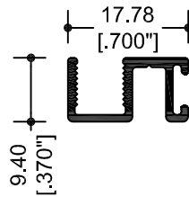
20572 CERCÓ Y ZOCLO
