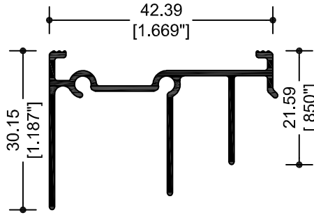
10568 CABEZAL
