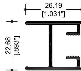
7107 CERCO FIJO
