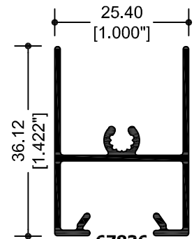
67836 CABEZAL VENTANA
