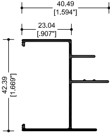
10570 JAMBA
