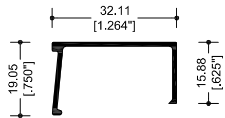
9112 JUNQUILLO
