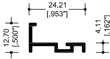
67013 BASE
