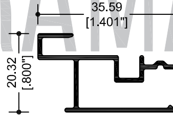
19272 TRASLAPE
