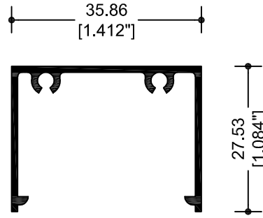
29076 BOLSA LISA
