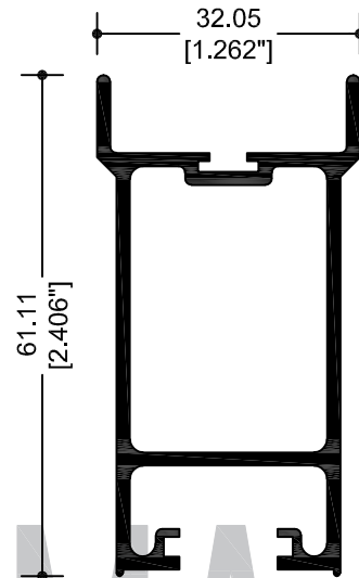
67850 CERCO OXXO
