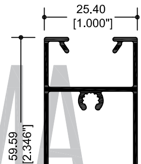
67836 CABEZAL VENTANA
