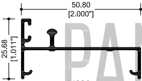
14286 RIEL
