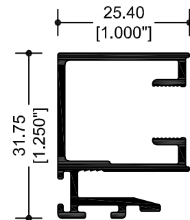
7106 CERCO TRASLAPE
