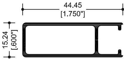
67821 CERCO PUERTA
