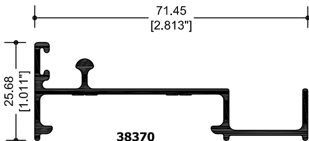
38370 RIEL CON MOSQ. EXT
