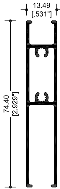
37825 ZOCLO PUERTA
