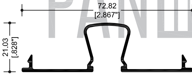
67315 TAPA BOLSA
