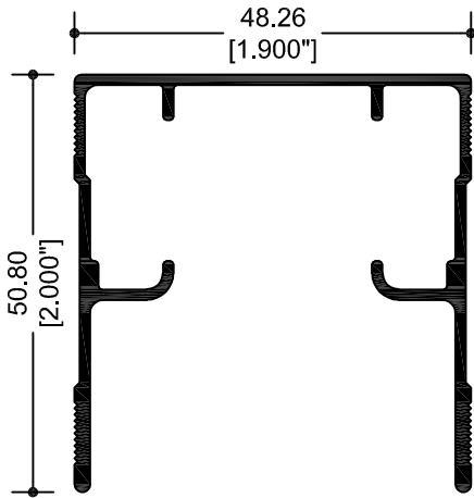
9947 RIEL SUPERIOR
