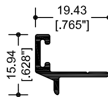
10220 ADAPTADOR OXXO
