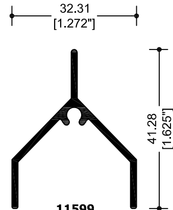
11599 REJILLA
