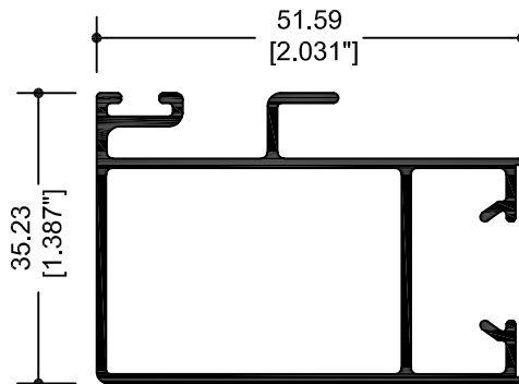
67848 TRASLAPE PUERTA
