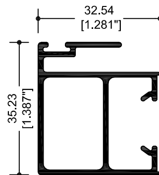
67844 CERCO TRASLAPE VENTANA
