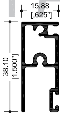
10358 MOSQUITERO
