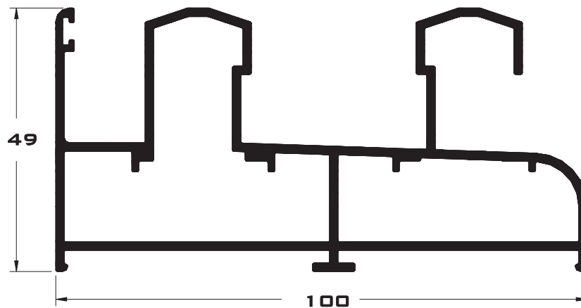
10002 CERCO PERIMETRAL
