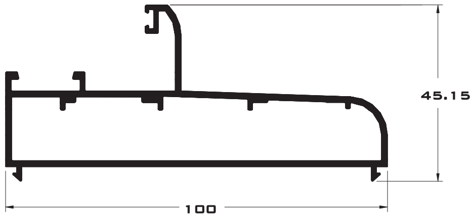
10003 FIJO TUBULAR
